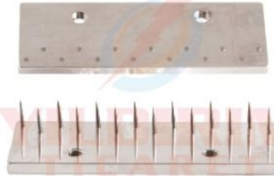
Speretto Ram İğnesi 14'lü Sperotto Stenter Pin Plate - 14 pins
