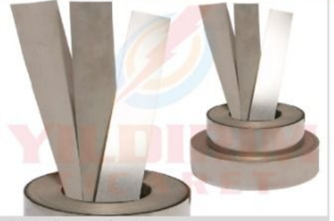
Ragle Sıyırma Bıçakları (0,15x40-0,15x45-0,15x30-0,15x33-0,15x50-0, 15x55-0,20x45-0,20x50-0,20x55) Squeegee Blade Rolls
