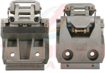
Brückner Ram Mandalı Saçlı Bruckner Combined Pin Clip
